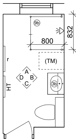
Typ 1b med dusch
