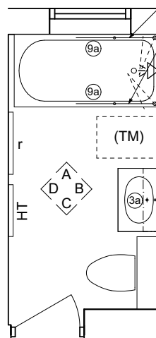
Typ 1b med badkar
